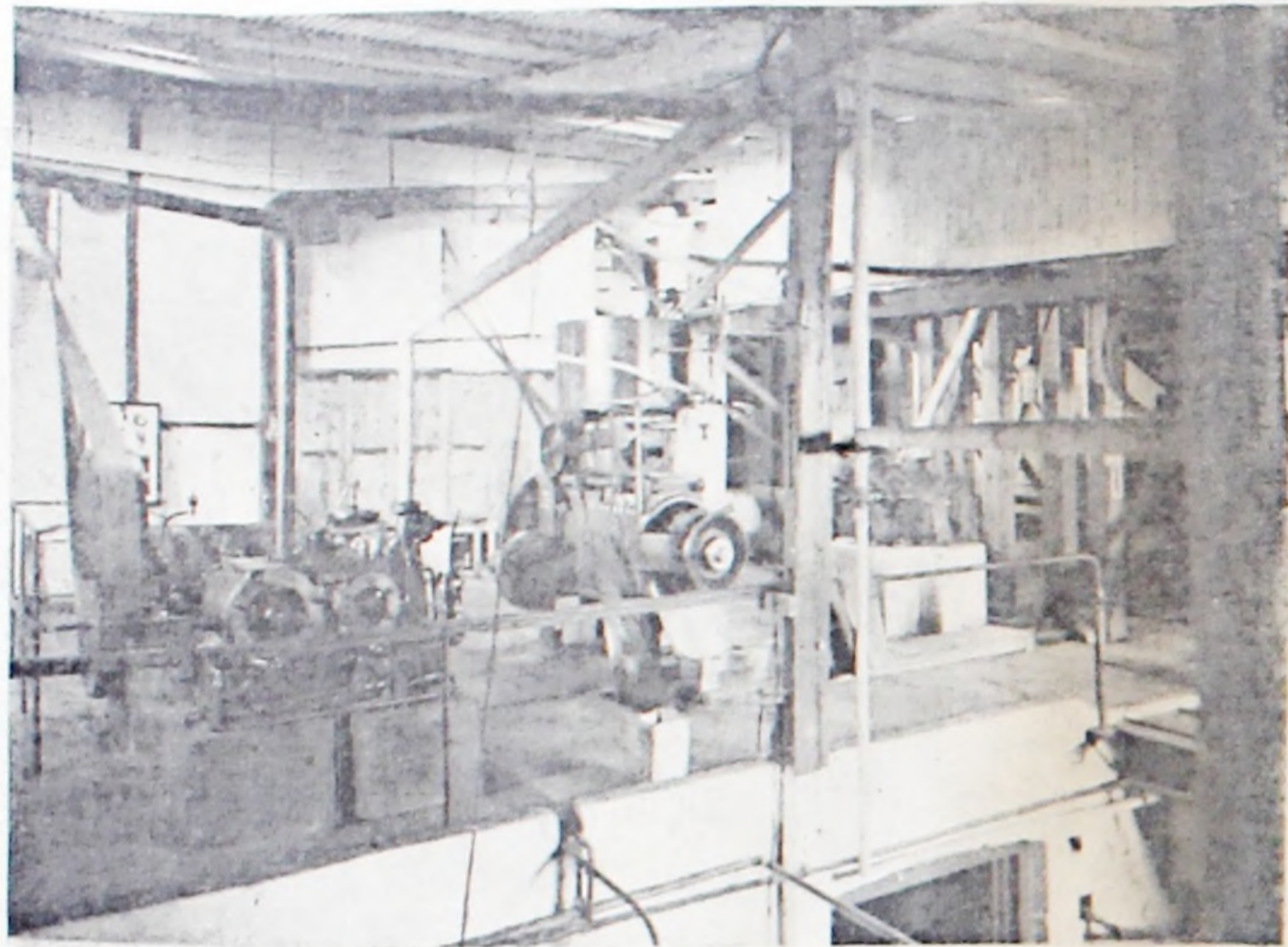
La modernísima prensa recientemente adquirida, en Alemania y una parte de los elevadores existentes en el piso superior de este importante establecimiento.
