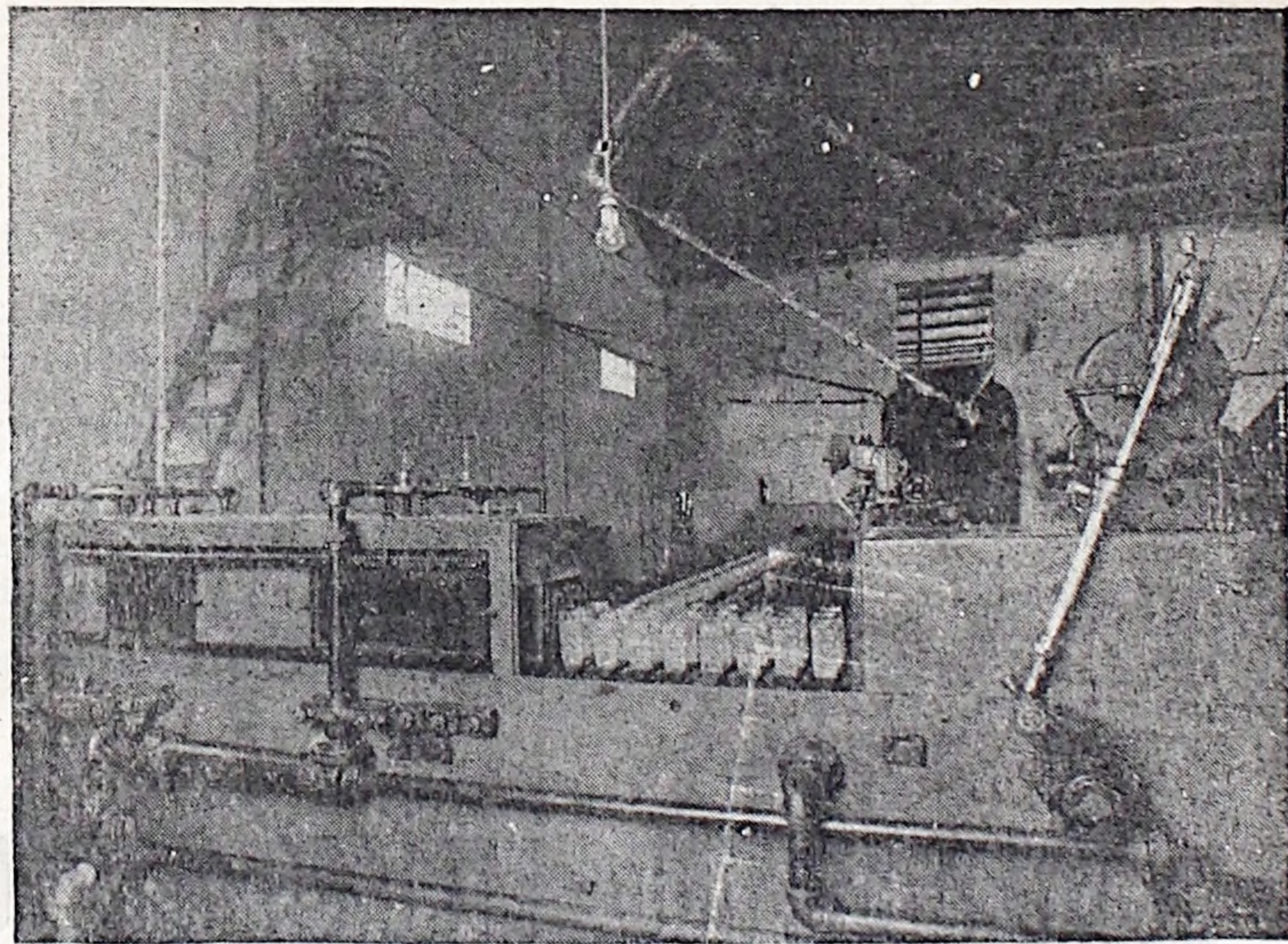
Lavadora y esterilizadora de botellas "DIXIE"
