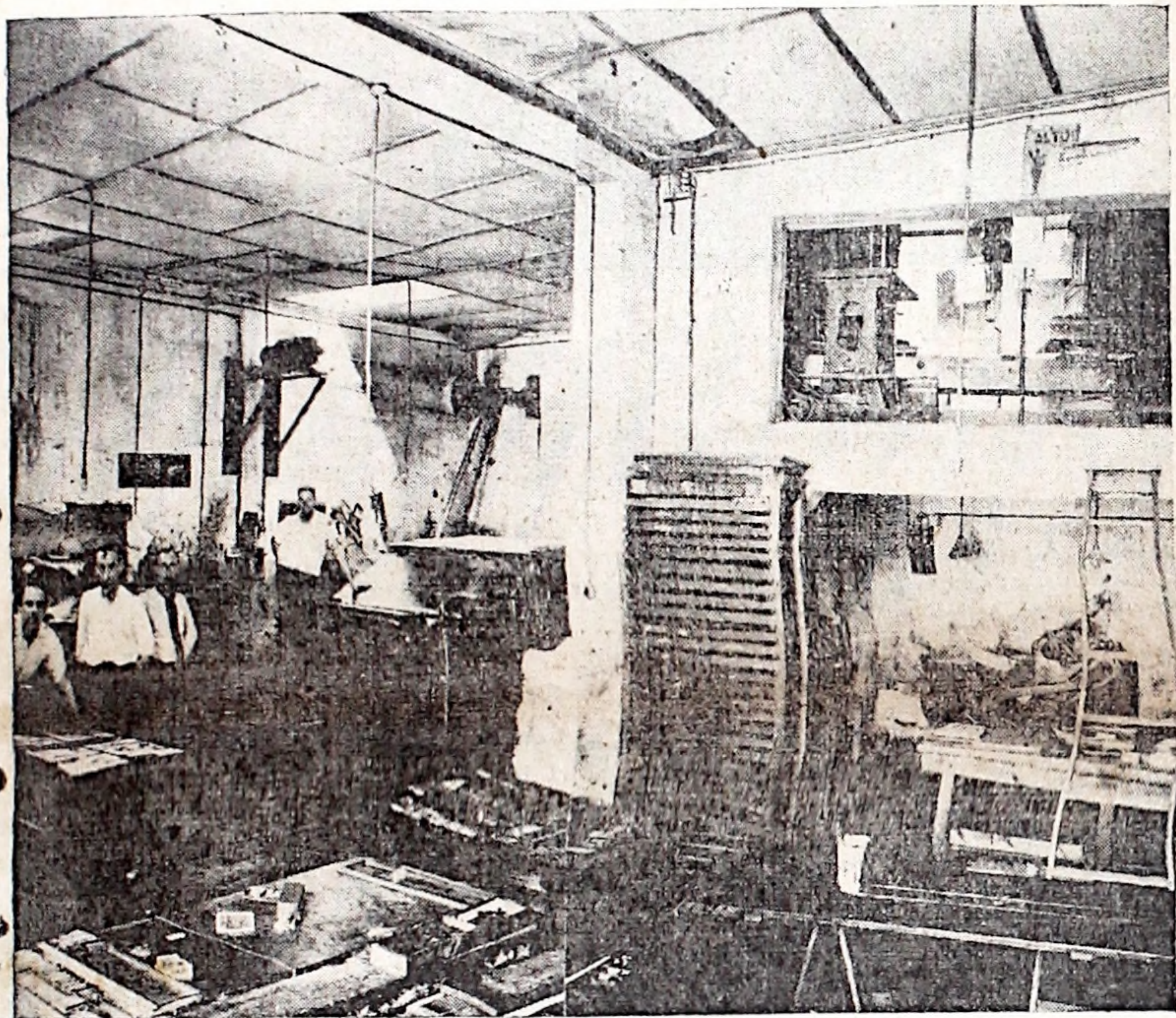
Aspecto parcial de los talleres gráficos de TRIBUNA SALTEÑA, tomado en un alto de la jornada de todos los días. — A la derecha del lector, en ángulo superior, parte de la máquina y taller de fotograbados. — Debajo, minerva y sección de tipografía. — La otra nota, corresponde a nuestra máquina impresora e instrumentales diversos de la confección del diario.
