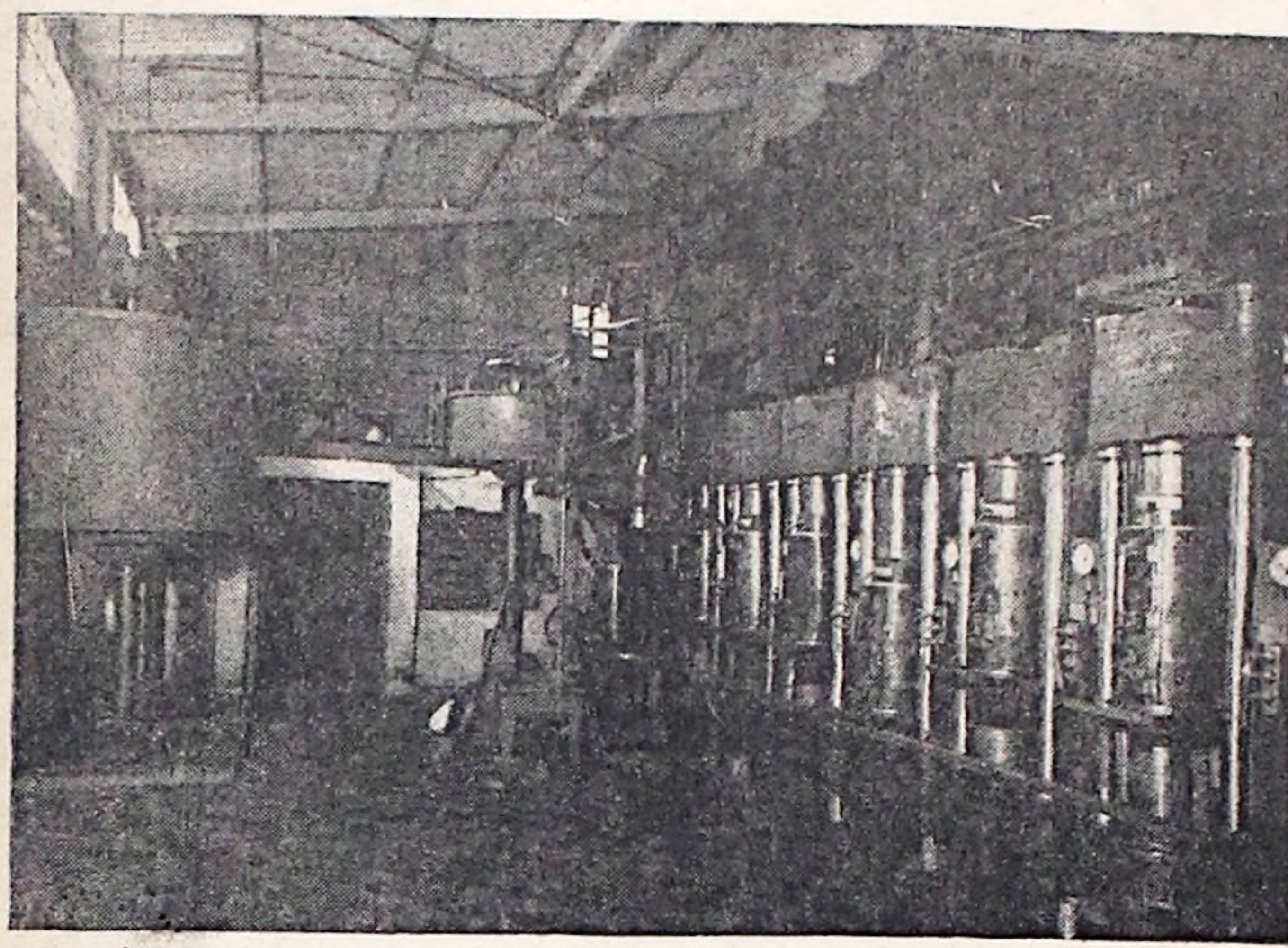
Prensas hidráulicas que se utilizan en la fábrica de aceite.
